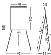
A 711/N 185 100 x 70 0,5
