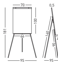
B 704/N 181 100 x 70 0,5
